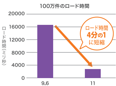
pgbench_accounts テーブルを10万件ずつ10個のテーブルに範囲パーティショニングで分割した場合
